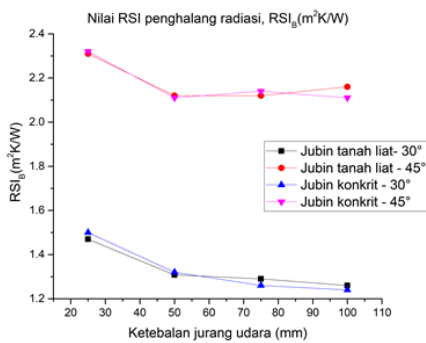
RAJAH 6. Nilai RSI sistem penghalang radiasi untuk pelbagai ketebalan jurang udara reflektif
