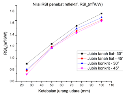
RAJAH 5. Nilai RSI sistem penambat reflektif untuk pelbagai ketebalan jurang udara reflektif
