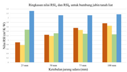
RAJAH 8. Ringkasan nilai RSI_A dan RSI_B untuk bumbung jubin tanah liat
