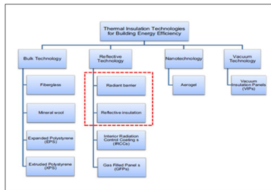
RAJAH 1. Klasifikasi bahan penebat (Lee et al. 2016)
