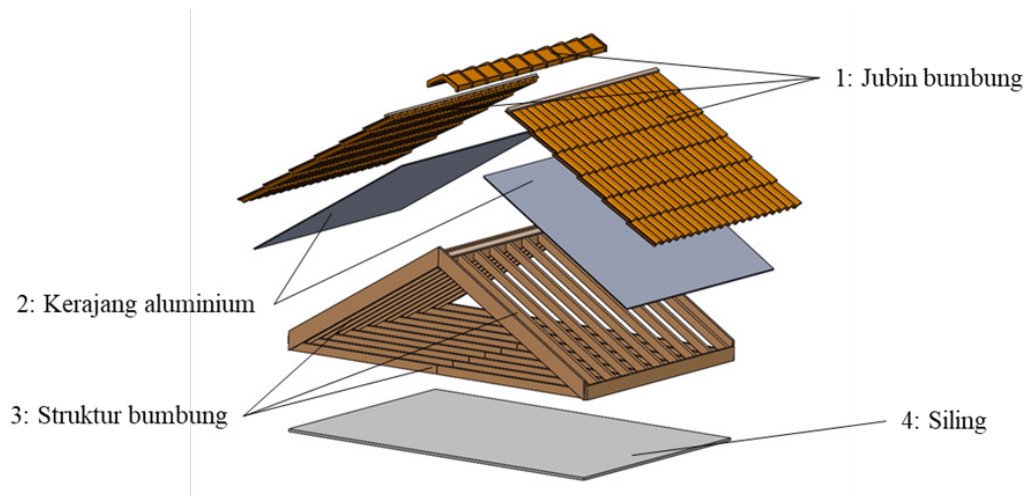
RAJAH 4. Pandangan besar bumbung yang menggabungkan sistem penebat reflektif dan sistem penghalang radiasi (1: Jubin bumbung; 2: Kerajang bumbung; 3: Struktur bumbung; 4: Siling)
