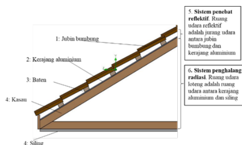
RAJAH 2. Padangan rentang lintang bumbung yang menggabungkan sistem penambat reflektif dan sistem halangan radiasi
