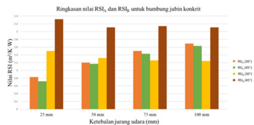
RAJAH 9. Ringkasan nilai RSI_A dan RSI_B untuk bumbung jubin konkrit
