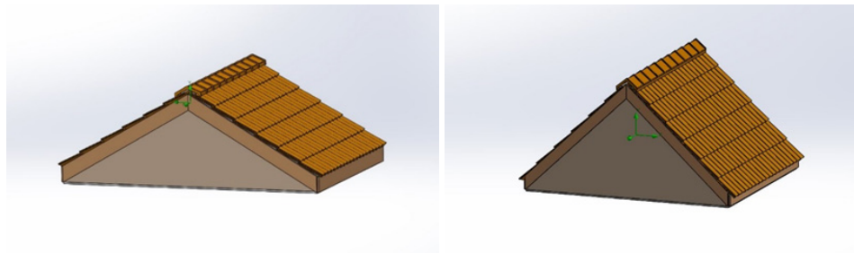
RAJAH 3. (i) Bumbung bersudut 30°. (ii) Bumbung bersudut 45°
