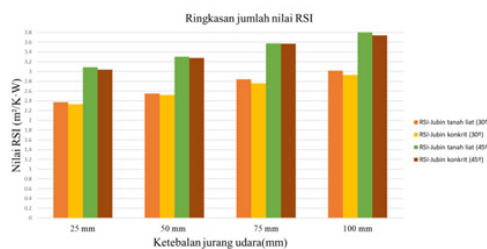
RAJAH 10. Jumlah nilai RSI untuk semua konfigurasi bumbung
