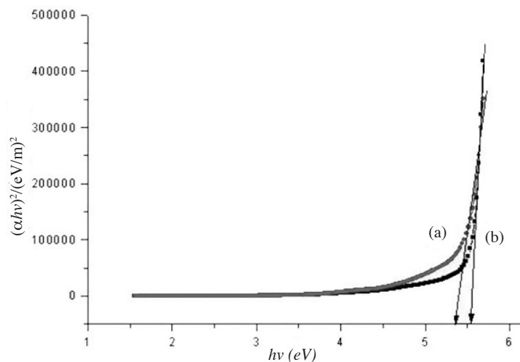
RAJAH 3. Graf (\alpha hv)^2 melawan hv untuk nanozarah zink oksida yang dieramkan selama (a) 2 jam dan (b) 18 jam. Unjuran memberikan nilai E_g = (a) 5.42 dan (b) 5.52 eV
