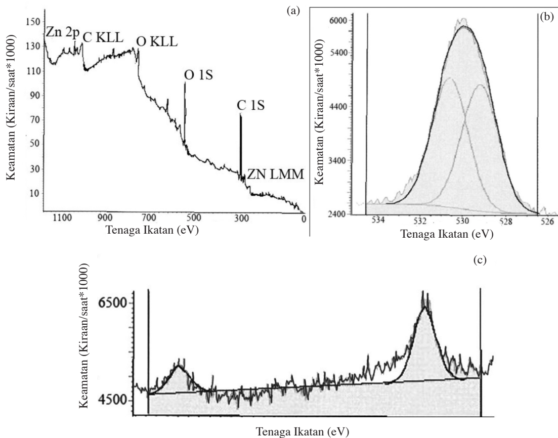
RAJAH 6. (a) Spektrum lebar XPS bagi nanozarah zink oksida dengan masa penderaman 2 jam di dalam afrons gas koloid serta spektrum XPS resolusi tinggi bagi (b) teras O(1s) dan (c) teras Zn(2p)
