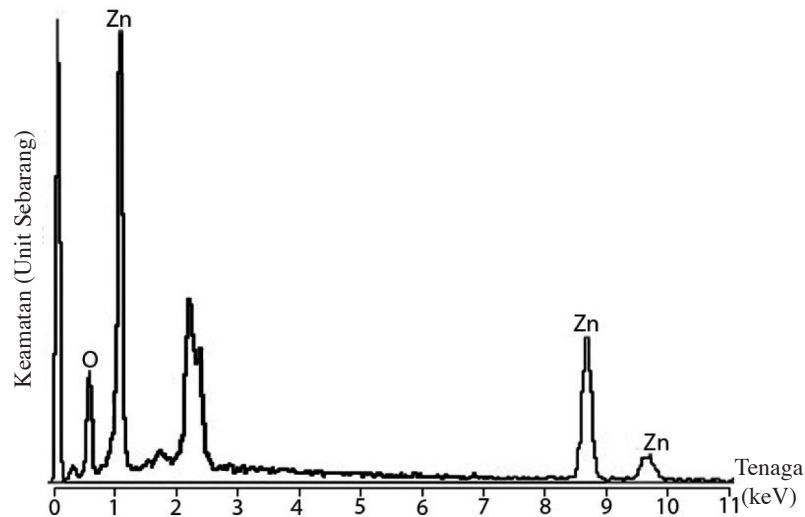
RAJAH 5. Corak graf analisis EDXA bagi 18 jam waktu penderaman yang menunjukkan kehadiran unsur-unsur karbon, zink, oksigen dan aurum
