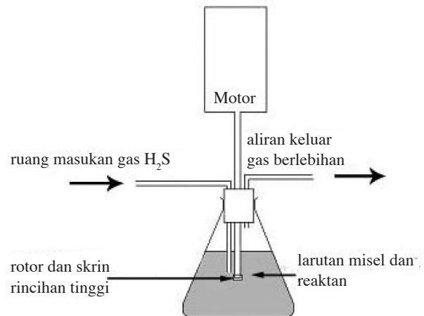
RAJAH 1. Susun atur reaktor nanozarah dan afrons gas koloid
