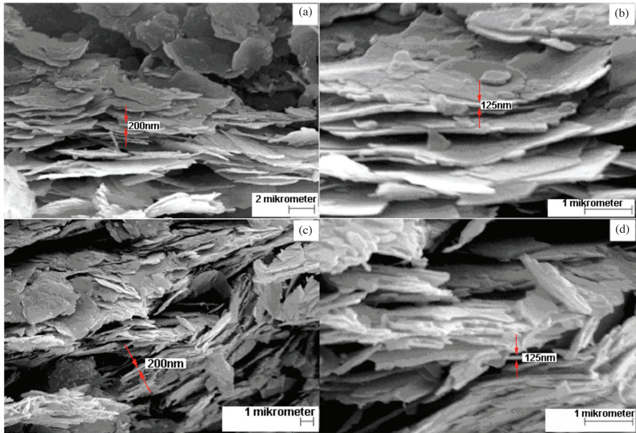
RAJAH 4. Mikrograf SEM bagi sampel zink oksida dengan 2 jam masa pengeraman di bawah (a) 4000 kali pembesaran dan (b) 15 000 kali pembesaran dan dengan 18 jam masa pengeraman di bawah (c) 4000 kali pembesaran dan (d) 15 000 kali pembesaran
