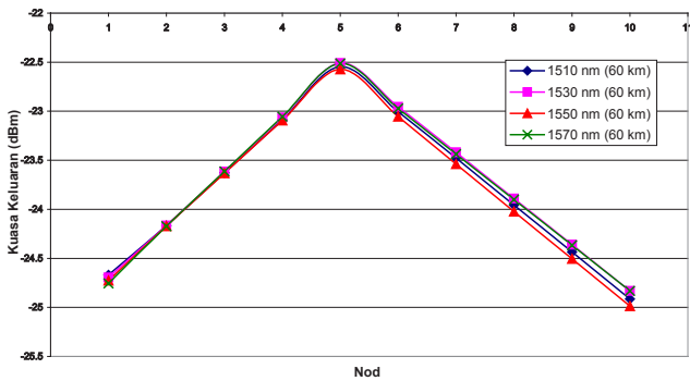
RAJAH 6. Penurunan pada Kuasa Lesapan Berlaku Sehingga Nod ke-5 dan Meningkatkan Semula Sehingga ke Nod ke-10 Disebabkan Gandaan Diturunkan Sebanyak 1 dB. Pengukuran Dijalankan pada OC-48 dan Jarak Antara Dua Nod 60 km
