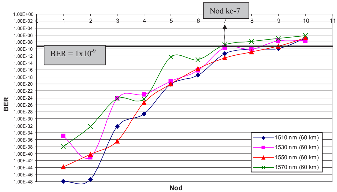
RAJAH 13. Kenaikan pada Nilai Ganda Pra Pertama Meningkatkan Mengurangkan Nilai BER untuk Nod Pertama dan Nilainya Meningkatkan untuk Nod yang Seterusnya. Nilai BER yang Kecil pada Permulaan Memberi Kesan yang Baik Terhadap Prestasi Keseluruhan Sistem
