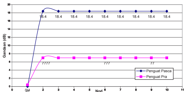
RAJAH 2. Gandaan Pascapenguat dan Prapenguat untuk Profil A. Nilai Gandaan Ini Bersamaan dengan Nilai Lesapan yang Dijanakan oleh Beban Talian
