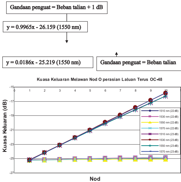
RAJAH 17. Penambahan 1 dB Melebihi Nilai Beban Talian pada Gandaan Penguat Memberi Kesan yang Besar Terhadap Kuasa Keluaran pada Setiap Nod. Perbandingan Dilakukan dengan Gandaan Penguat yang Menyamai Nilai Beban Talian yang Menghasilkan Profil Kuasa yang Malar. Kadar Penghantaran Data Adalah 2.5 Gbps
