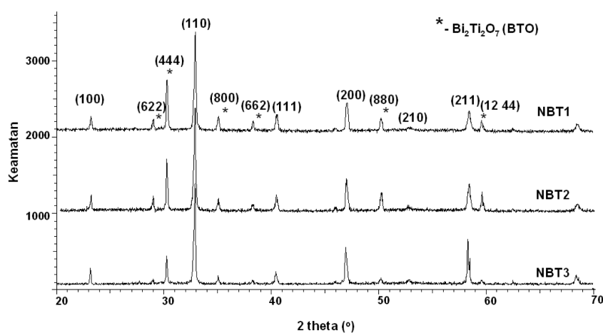
RAJAH 2. Difraktogram sinar-x bagi NBT yang disinter pada 3 suhu yang berlainan
